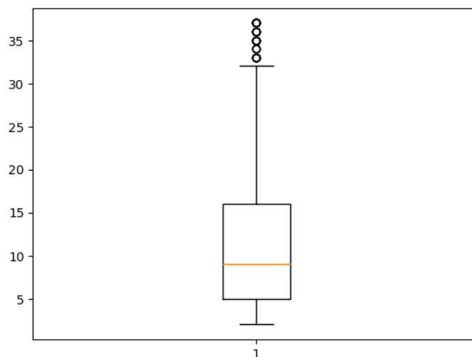
Рис. 2. Диаграмма размаха (boxplot) распределения реакций на постах Fig. 2. Boxplot of distribution of reactions on posts
